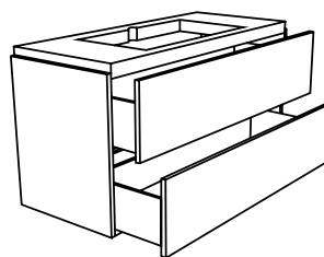
2 vonkajšie zásuvky v 2 úrovniach pod sebou š. 800 / 1000 / 1200 / 1400 mm
